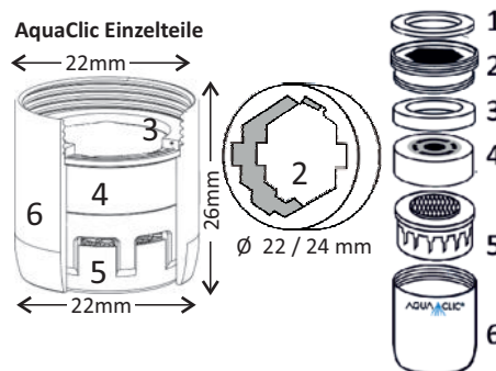
1 Adapter-Dichtung, 2 Universaladapter M22/M24, 3 Mengenregler mit Konstanthaltung, 5 Strahlregler mit Prallschutzkörper, 6 Metallhülse Edelstahl oder Messing mit bunter Kunststoffbeschichtung
